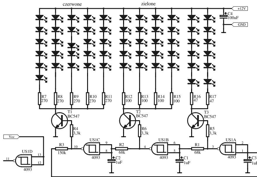
Schemat ideowy
