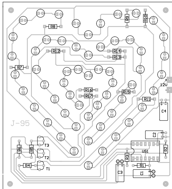
Schemat motażowy
